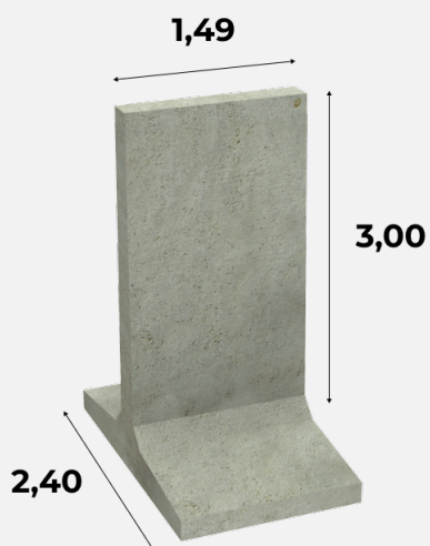
Typ 04 300x149x240 cm 5,035 t
