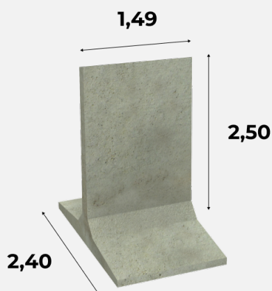
Typ 11 250x149x240 cm 3,306 t
