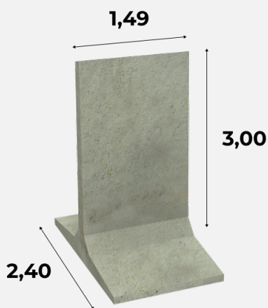
Typ 10 300x149x240 cm 3,580 t
