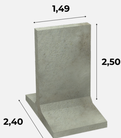
Typ 05 250x149x240 cm 4,593 t
