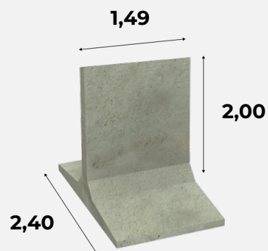
Typ 12 200x149x240 cm 3,007 t
