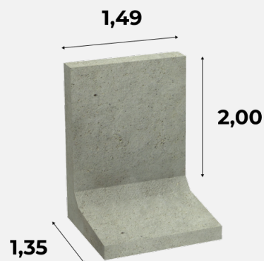
Typ 18 200x149x135 cm 3,119 t
